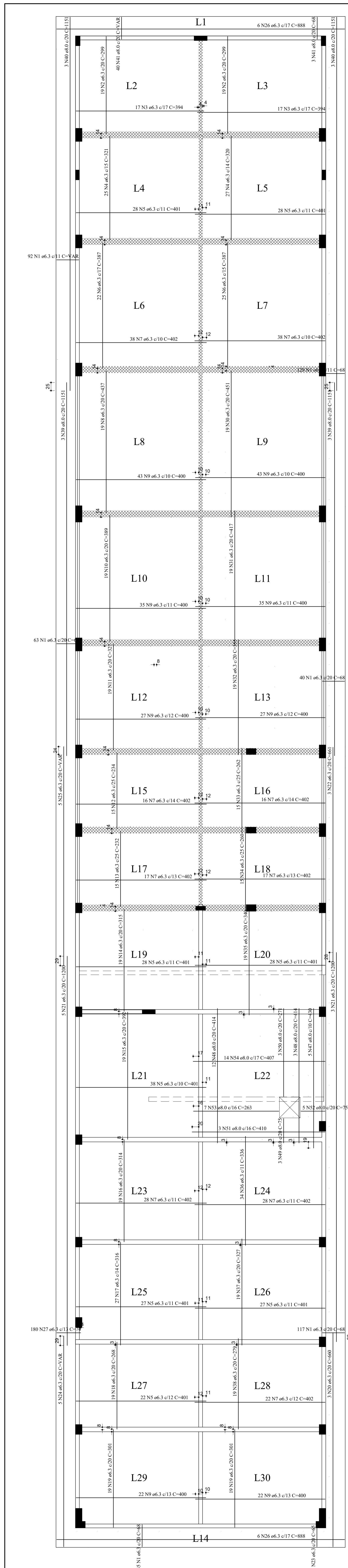
Armação positiva das lajes do pavimento 1º Pav. escala 1:50
